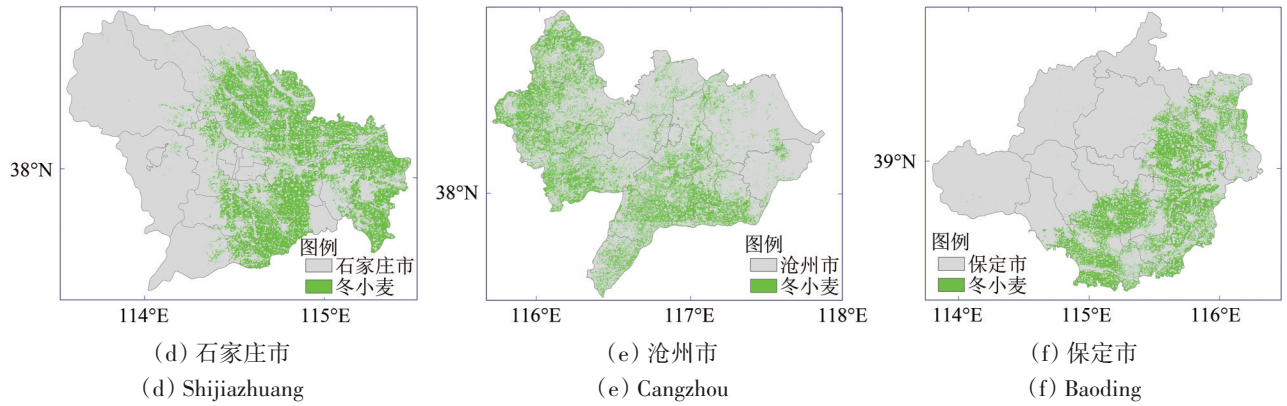
图 11 冬小麦提取结果图(市级)
